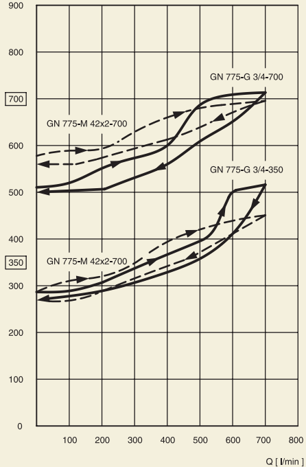
Druckverlauf \Delta p [mbar] im Behälter in Abhängigkeit vom Luftdurchsatz [l/min] bei Ventilöffnungsdruck 350 bzw. 700 mbar.
