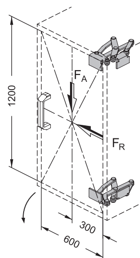
Standardtür für Dauertest
